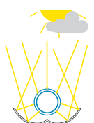
Diffuse Einstrahlung
