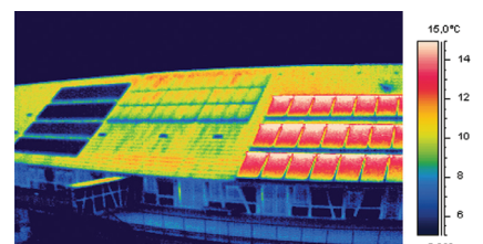
Thermographie | links: Paradigma Vakuumröhrenkollektoren, mitte: PV-Anlage, rechts: herkömmliche Flachkollektoren
